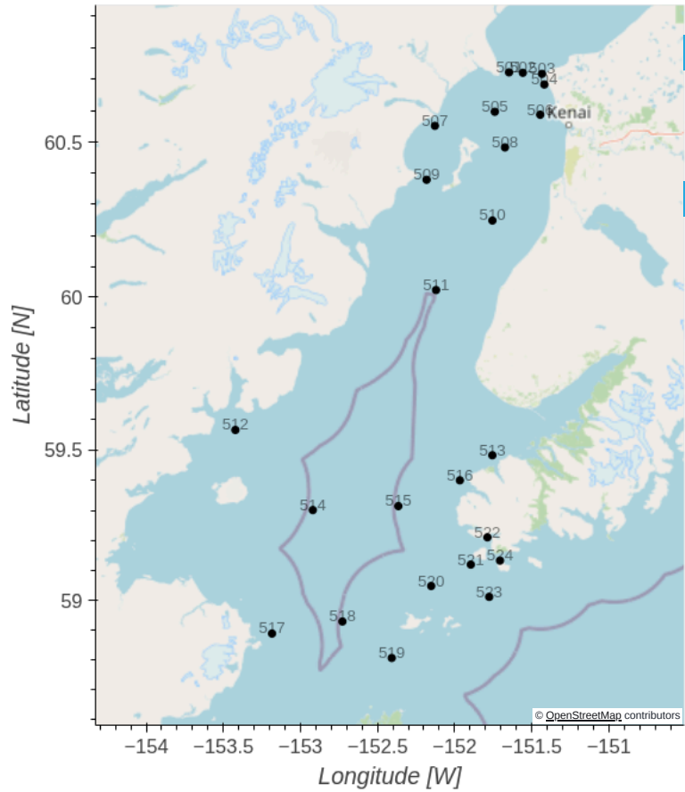
ctd_profiles_2005_noaa
